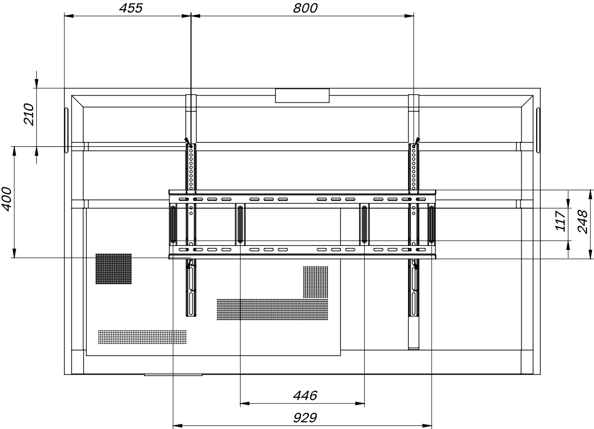
СХЕМА ПАНЕЛИ (ВИД СЗАДИ)
